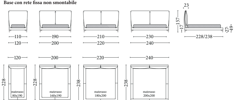
Base con rete fissa non smontabile
