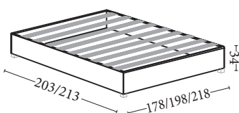
Base con rete fissa smontabile
