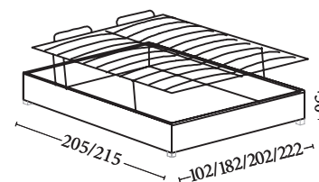
Base con rete sollevabile a due movimenti smontabile
