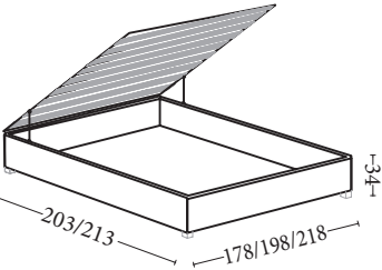
Base con rete sollevabile smontabile
